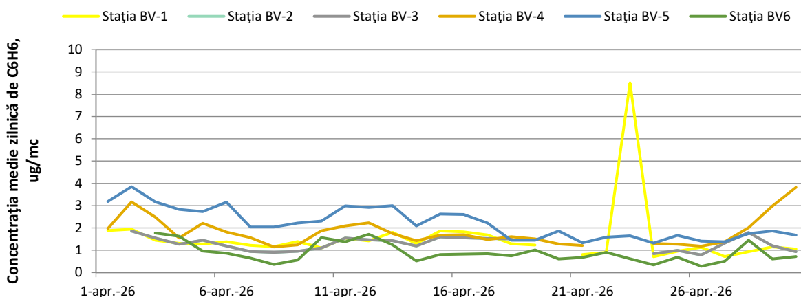
Figura 7. Evoluția concentrațiilor medii zilnice de benzen în luna aprilie 2026
