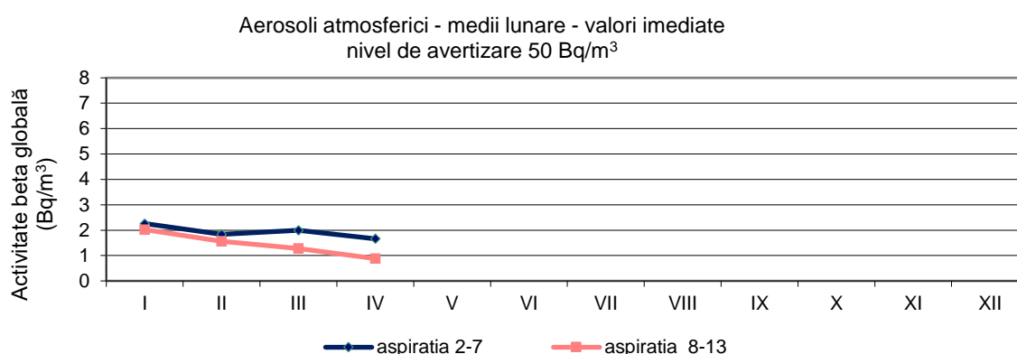
Figura 14. Activitatea beta globală pentru aerosoli atmosferici
