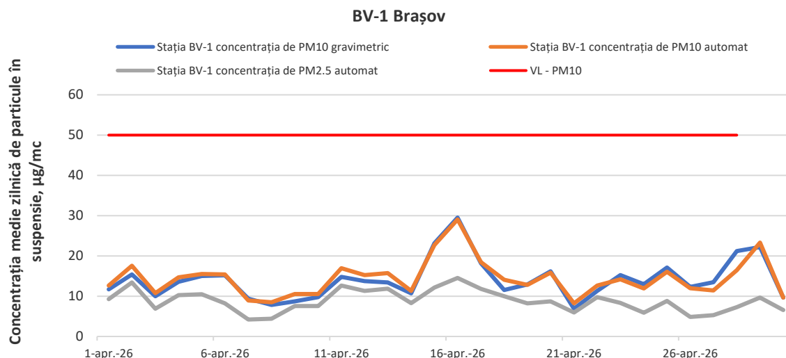
Figura 13. Evoluția concentrațiilor medii zilnice de PM10 gravimetric și automat și PM2,5 automat în stația de trafic BV-1, în luna aprilie 2026
