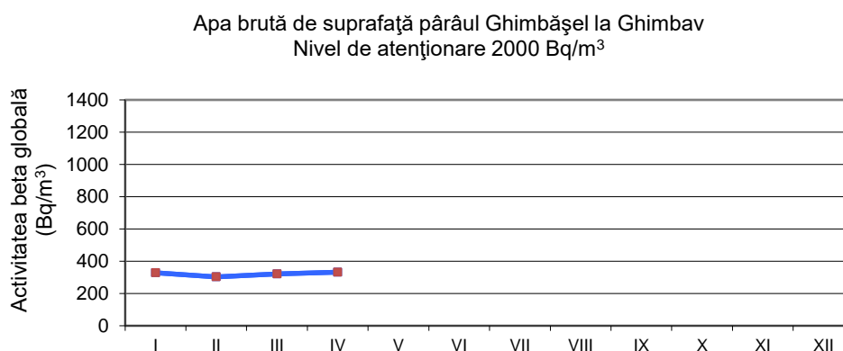
Figura 18. Activitatea beta globală imediată pentru apa de suprafață Pârâul Ghimbășel
