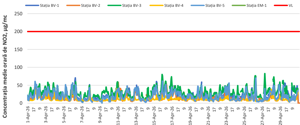
Figura 3. Concentrații medii orare de NO 2 în luna aprilie 2026
