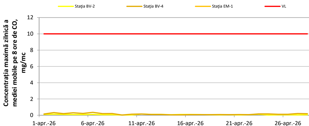
Figura 4. Concentrația maximă a mediei mobile pe 8 ore de CO în luna aprilie 2026
