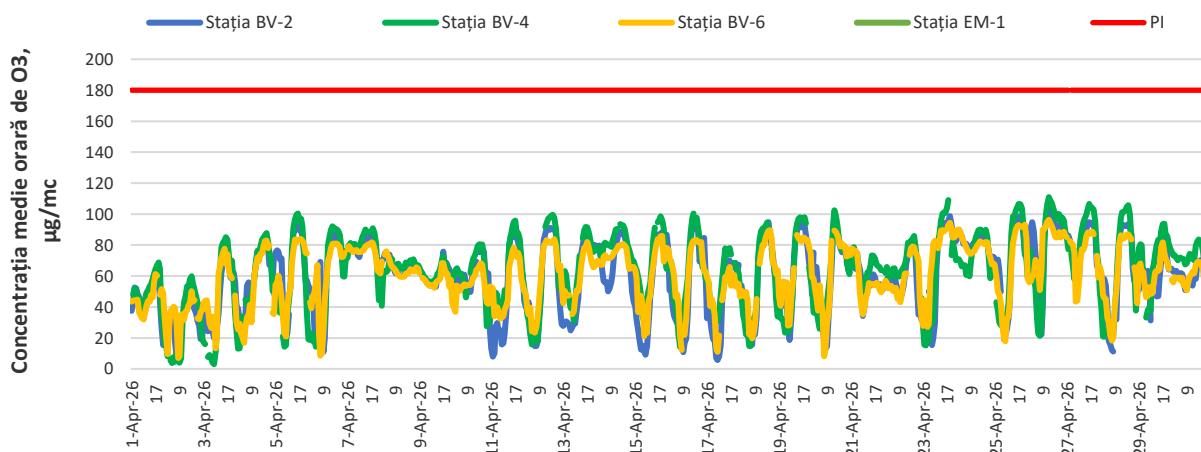
Figura 6. Evoluția concentrațiilor medii orare de O 3 în luna aprilie 2026
