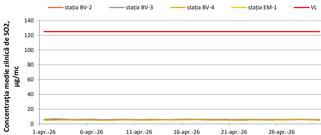
Figura 1. Evoluția mediilor zilnice de SO 2 în luna aprilie 2026
