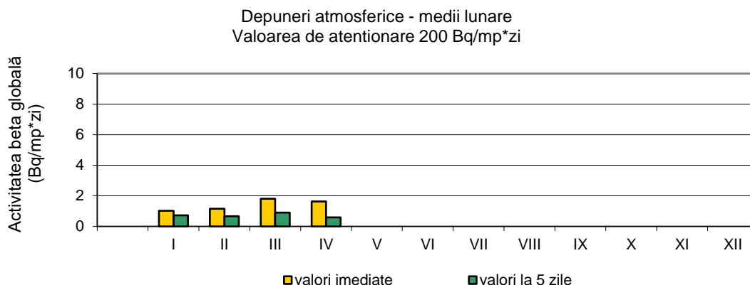
Figura 17. Activitatea beta globală pentru depuneri atmosferice
