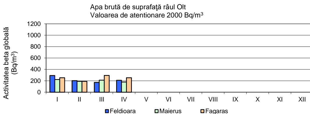
Fig. 20. Activitatea beta globală la 5 zile pentru apa de suprafață Râul Olt
