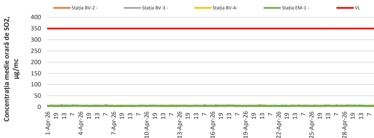
Figura 2. Evoluția mediilor orare de SO 2 în luna aprilie 2026
