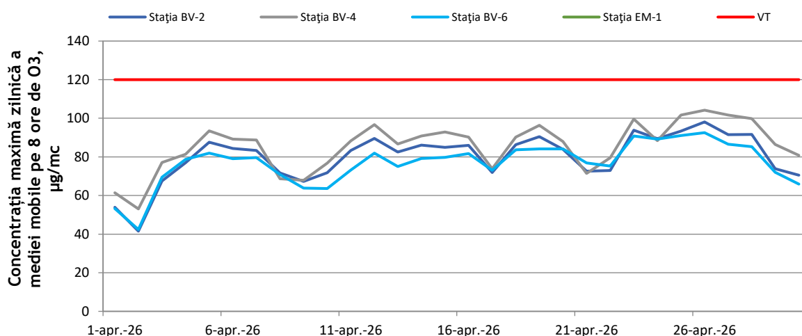
Figura 5. Evoluția concentrațiilor maximelor zilnice ale mediilor mobile pe 8 ore de O 3 în luna aprilie 2026
