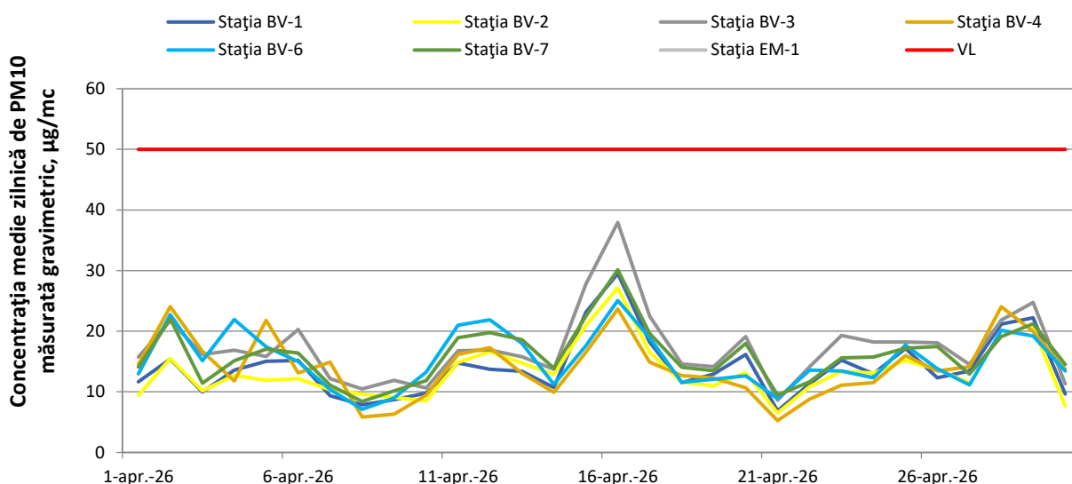
Figura 8. Evoluția concentrațiilor medii zilnice de PM10 (gravimetric) în luna aprilie 2026
