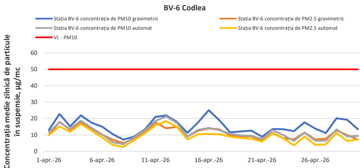
Figura 12. Evoluția concentrațiilor medii zilnice de PM10 gravimetric și automat și PM2,5 gravimetric și automat în stația de fond urban BV-6, în luna aprilie 2026
