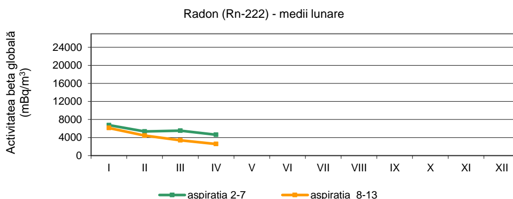
Figura 15. Activitatea calculată a Radonului
