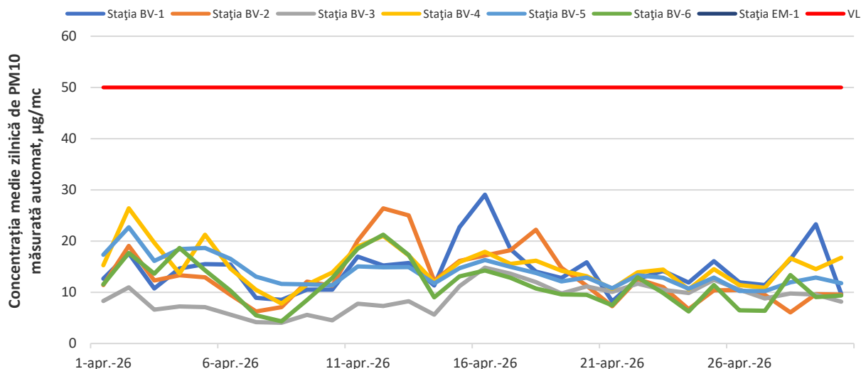
Figura 10. Evoluția concentrațiilor medii zilnice de PM 10 automat în luna aprilie 2026
